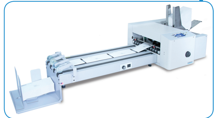
Optional AP-05 3-foot conveyor/stacker
